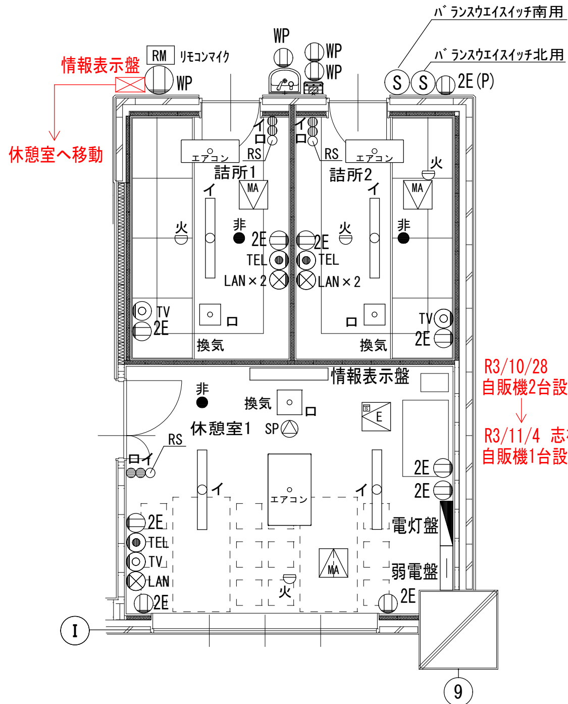
休憩室1・詰所2(詰所1) 平面図 (1/30)
