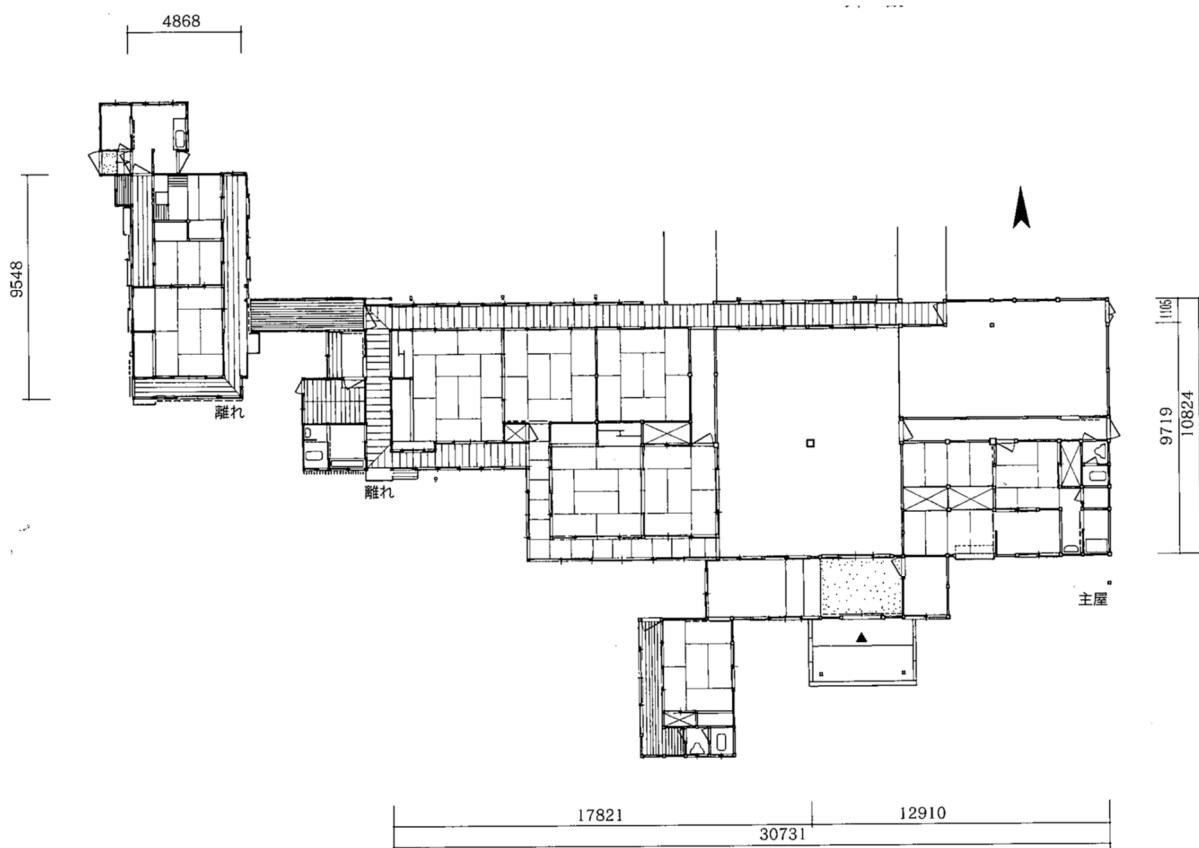
(別添4) 有隣荘庭園既存建物平面図 (CAD データなし)
