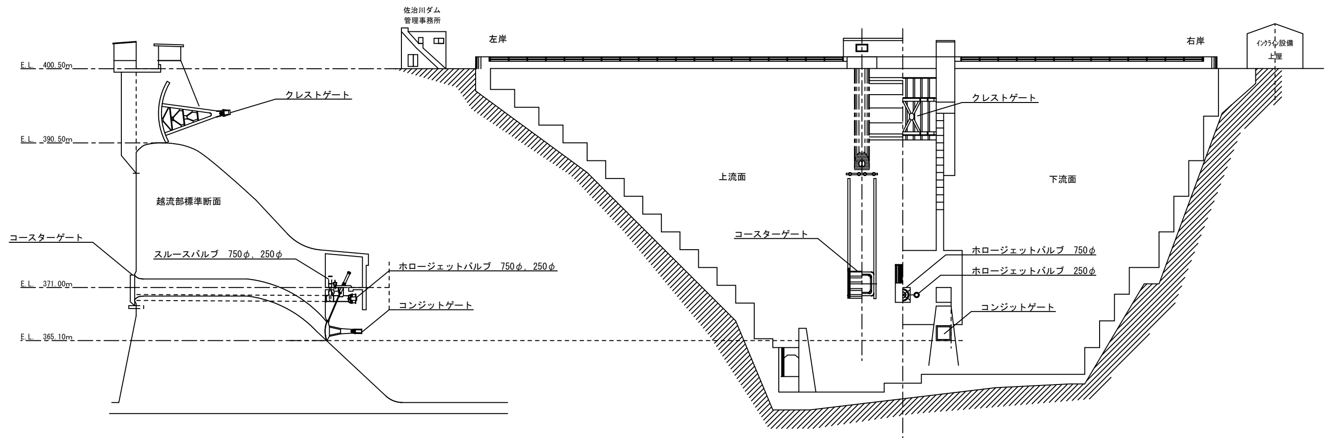
機器配置図
