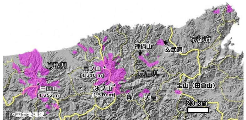
図1 鳥取県中・東部、兵庫県北部、京都府北部のおよそ1200万年前以降の火山岩の分布
