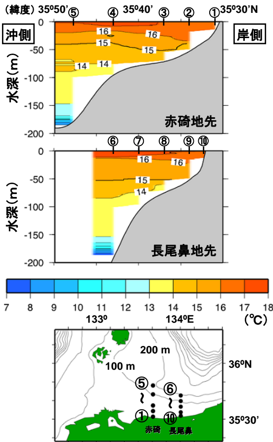
図1) 5月25日の赤碕と長尾鼻の地先における水温の鉛直分布(上図)と観測点(下図)。
