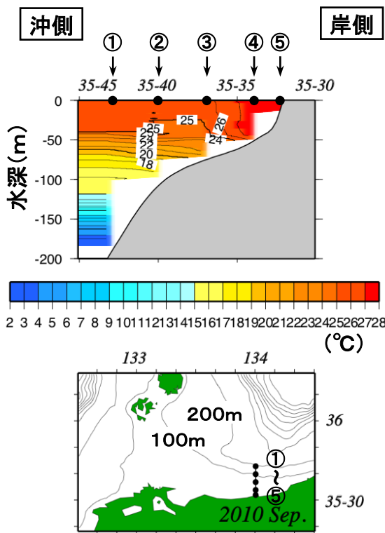
図1) 9月27日の水温の鉛直断面図
