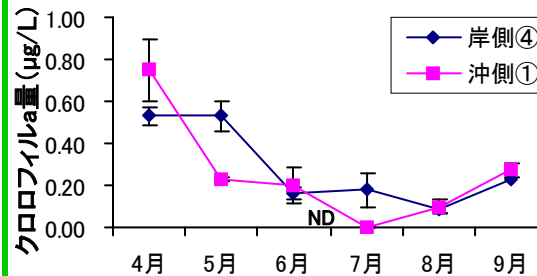
図3) 4~9月の20m以浅のクロロフィルaの平均値の変化。ND: 検出限界以下。
