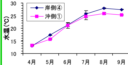
図2) 4~9月の20m以浅の水温の平均値の季節変化。
