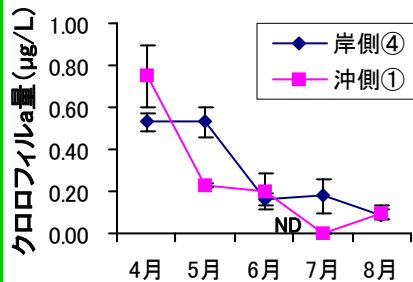
図3) 4～8月の20m以浅のクロロフィルaの平均値の変化。ND: 検出限界以下。
