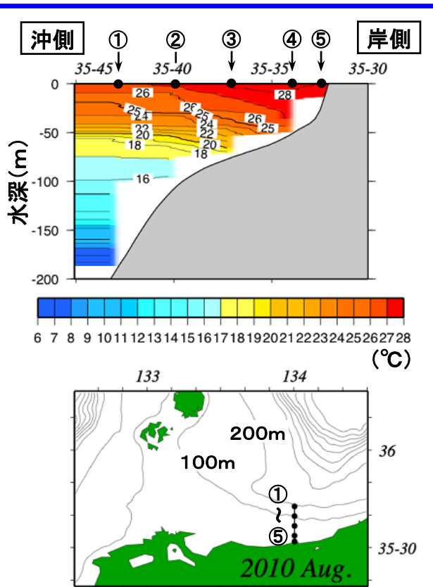
図1) 8月19日の水温の鉛直断面図
