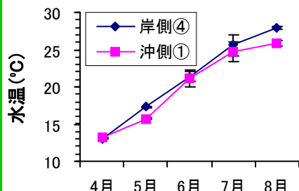
図2) 4～8月の20m以浅の水温の平均値の季節変化。
