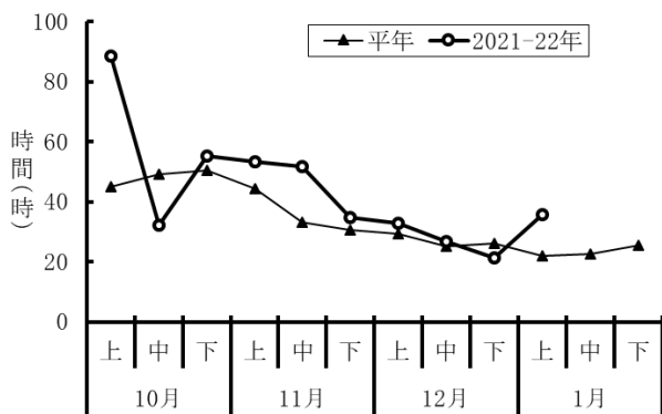
図3 2021-22年旬別日照時間(倉吉市)
