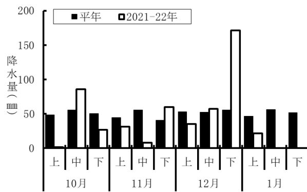
図4 2021-22年旬別降水量(倉吉市)
