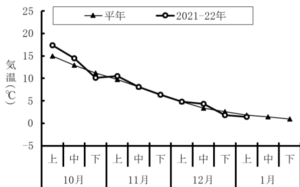
図2 2021-22年日最低気温(倉吉市)
