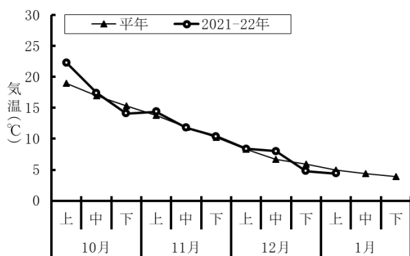
図1 2021-22年日平均気温(倉吉市)
