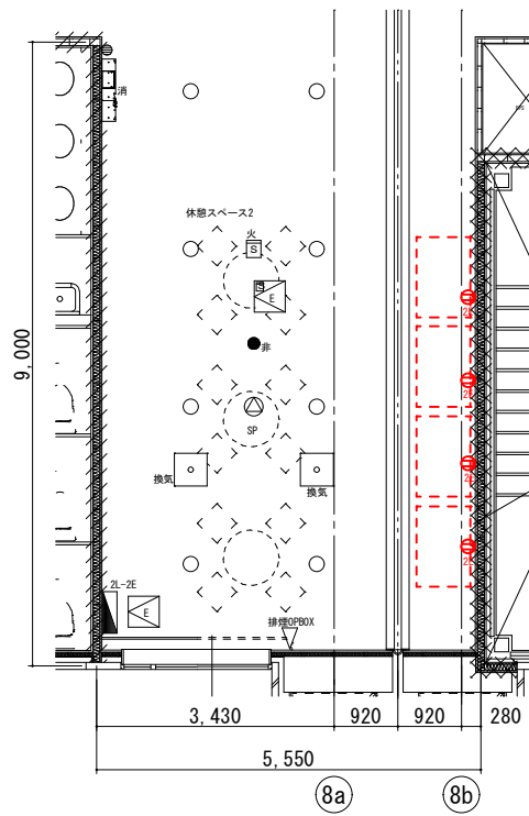
休憩スペース2 平面図 (1/60)
