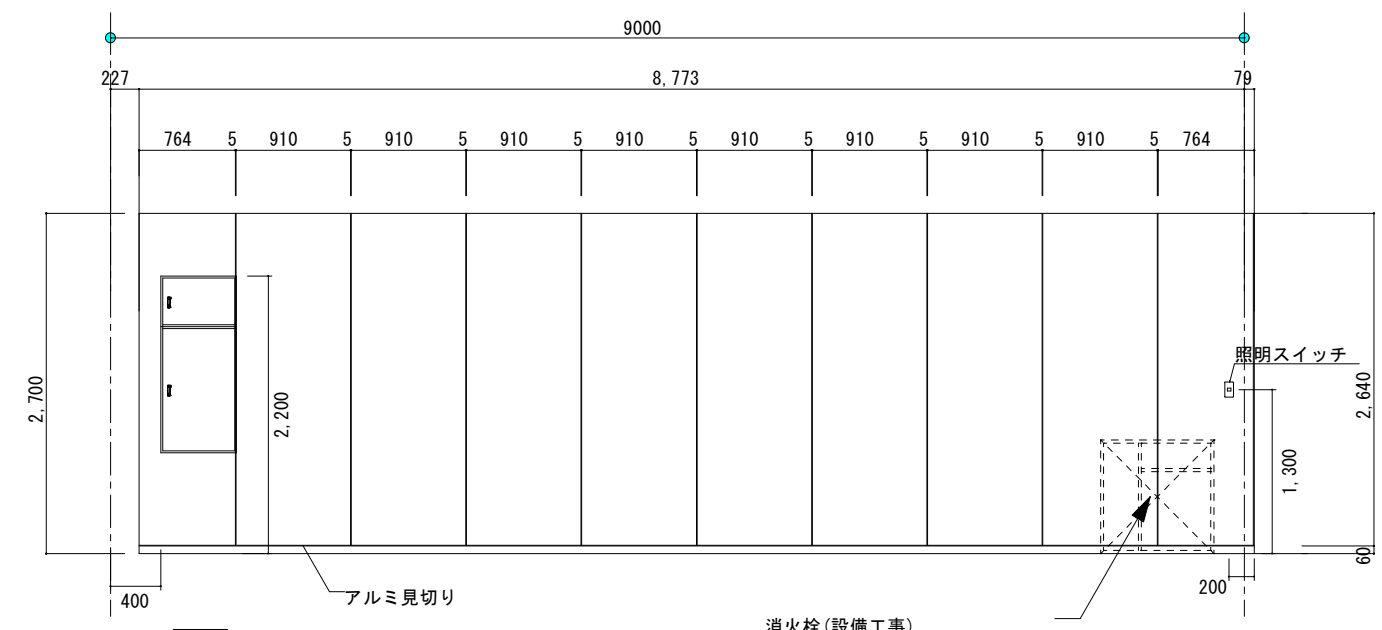
南面
