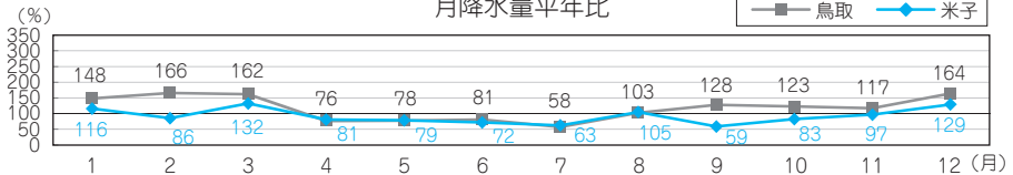
月降水量平年比
