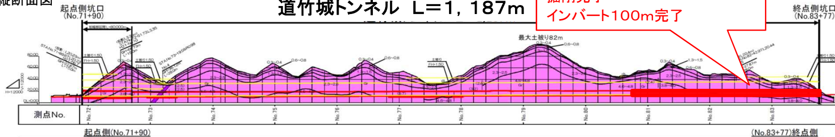
トンネル縦断面図
