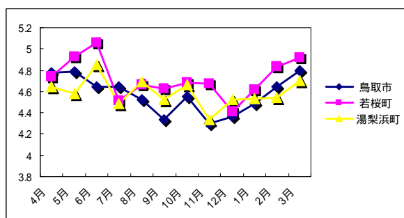
図1 平成20年度における pH の経月変化
