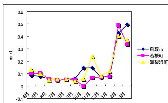
図4 平成20年度における nss-Ca 2+ 濃度の経月変化
