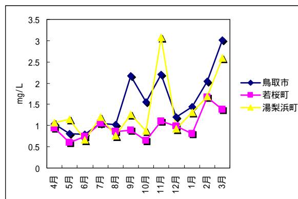
図3 平成20年度における NO 3 - 濃度の経月変化
