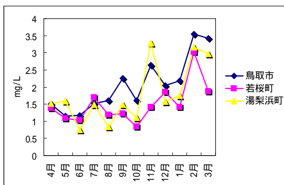
図2 平成20年度における nss-SO 4 2- 濃度の経月変化
