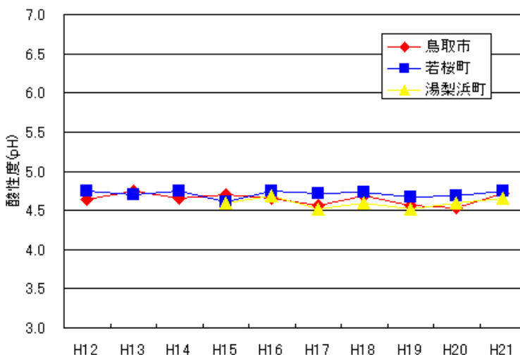
鳥取県における雨水のpH
