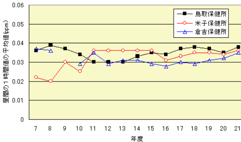
光化学オキシダント年平均値
