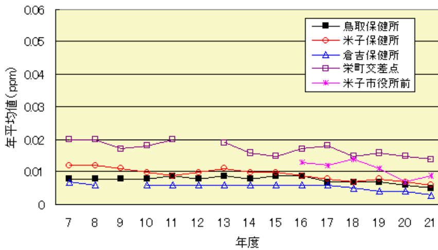
二酸化窒素の年平均値
