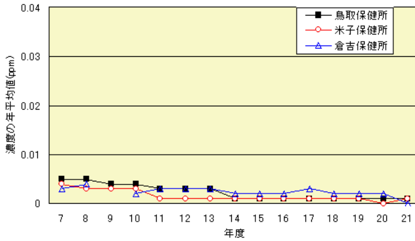
二酸化いおうの年平均値(一般環境大気測定局)
