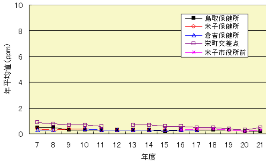
一酸化炭素の年平均値
