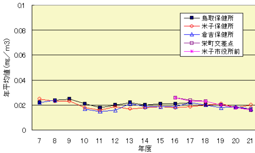
浮遊粒子状物質の年平均値
