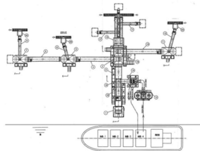
平面配置図
