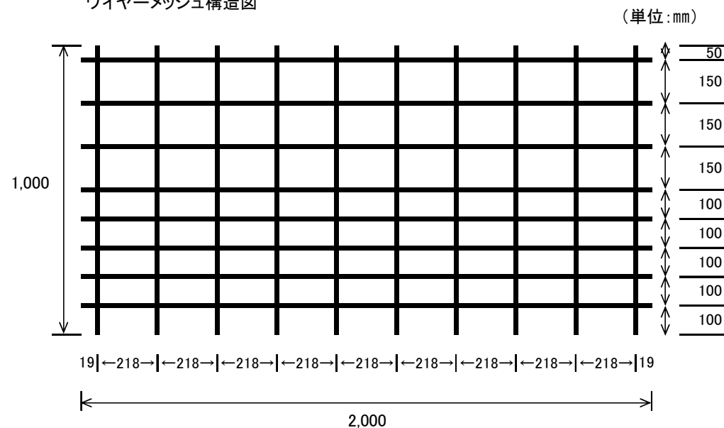
ワイヤーメッシュ構造図
