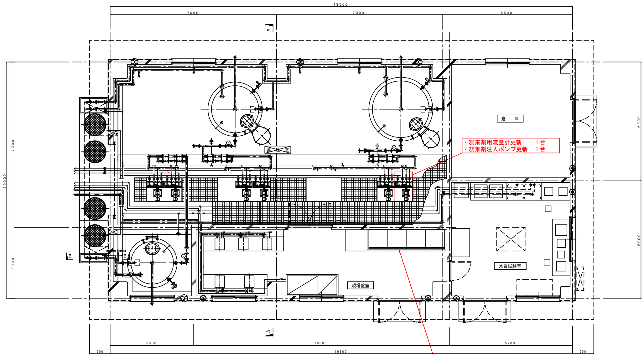
薬注棟平面図 S=1/50
