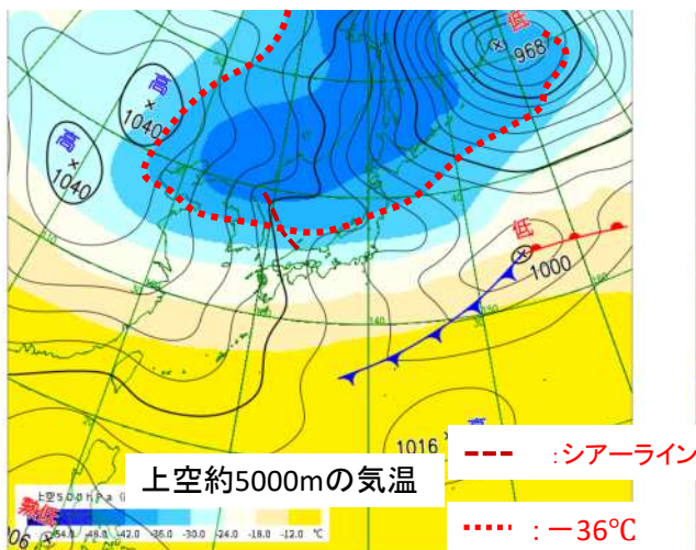
2月7日21時の予想天気図
