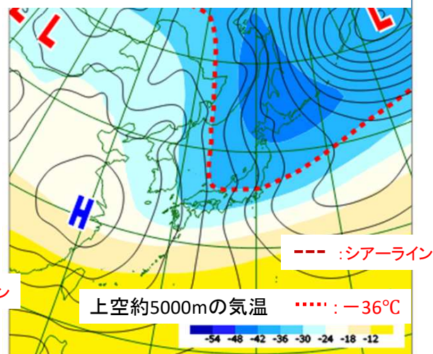
2月8日21時の予想天気図
