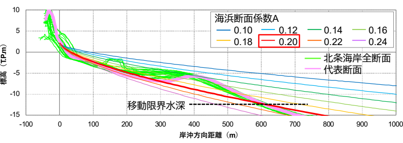
汀線後退量算定の代表断面
