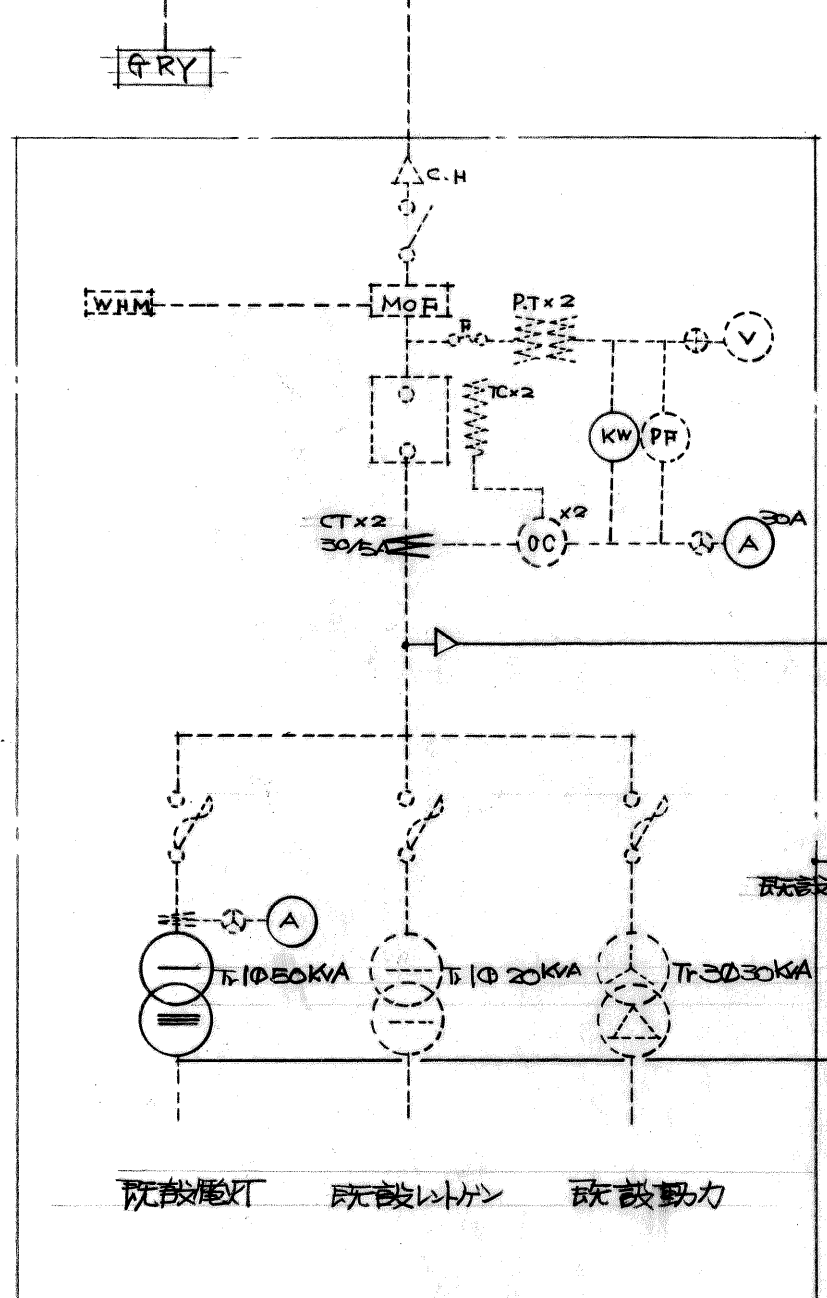
既設屋外キュービクル
