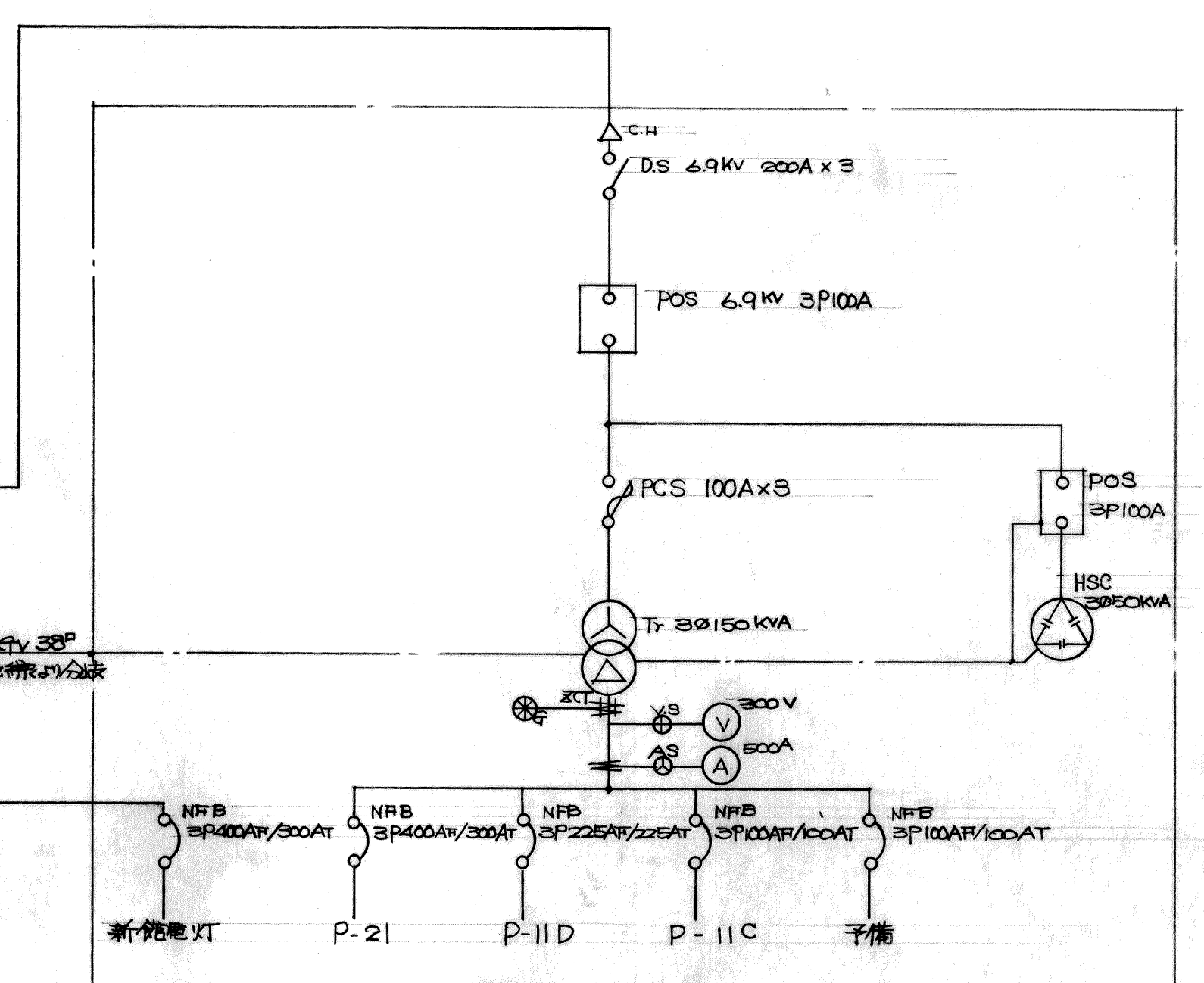
増設屋外キュービクル
