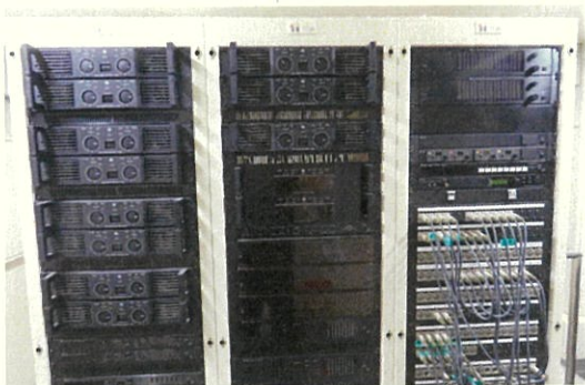
放送室 放送アンプ 全体
