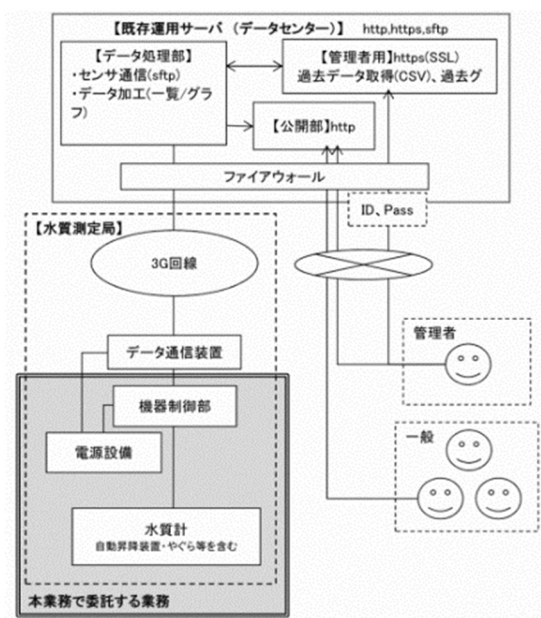
システム系統図
