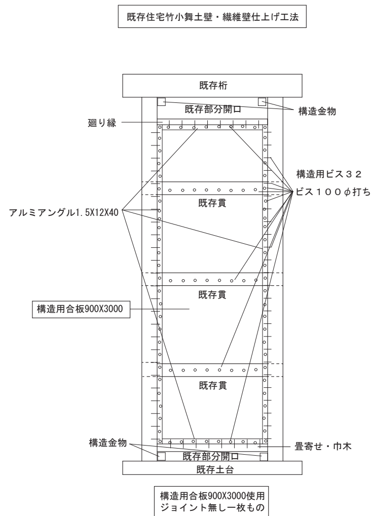
試験体仕様 1
