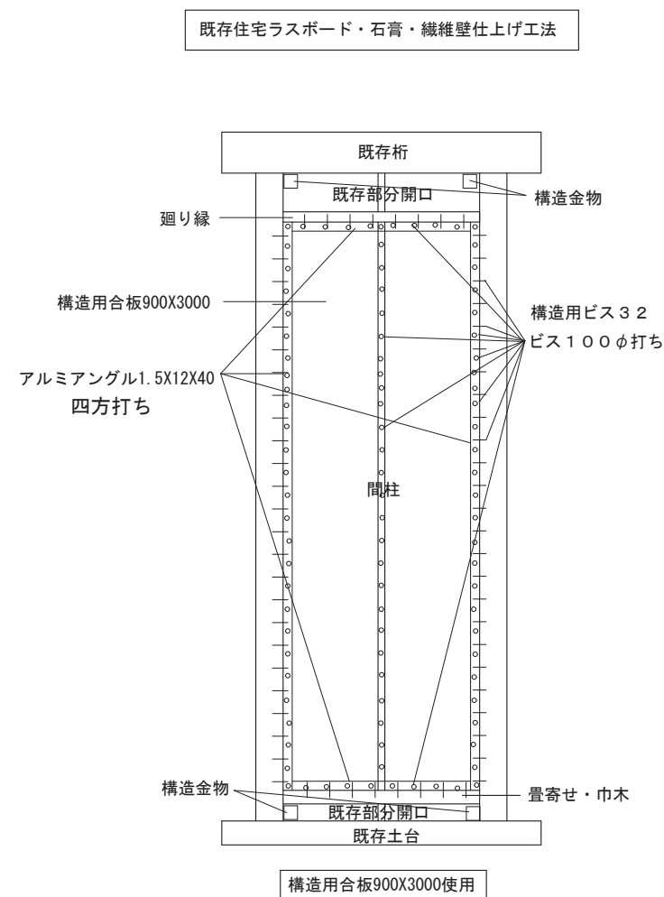
試験体仕様 3
