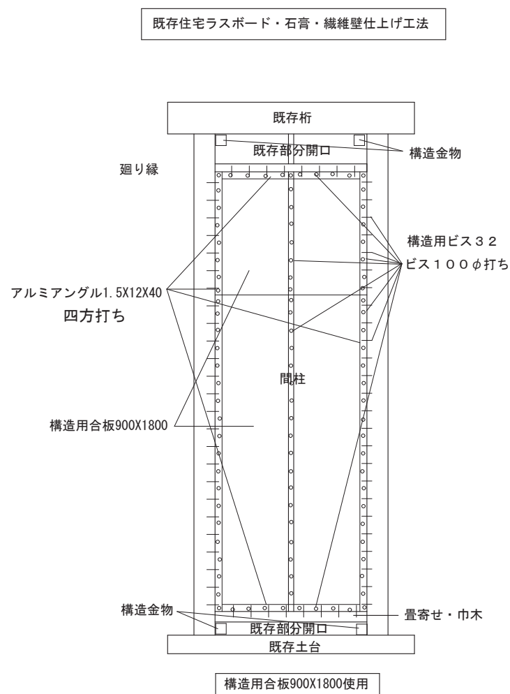
試験体仕様 2
