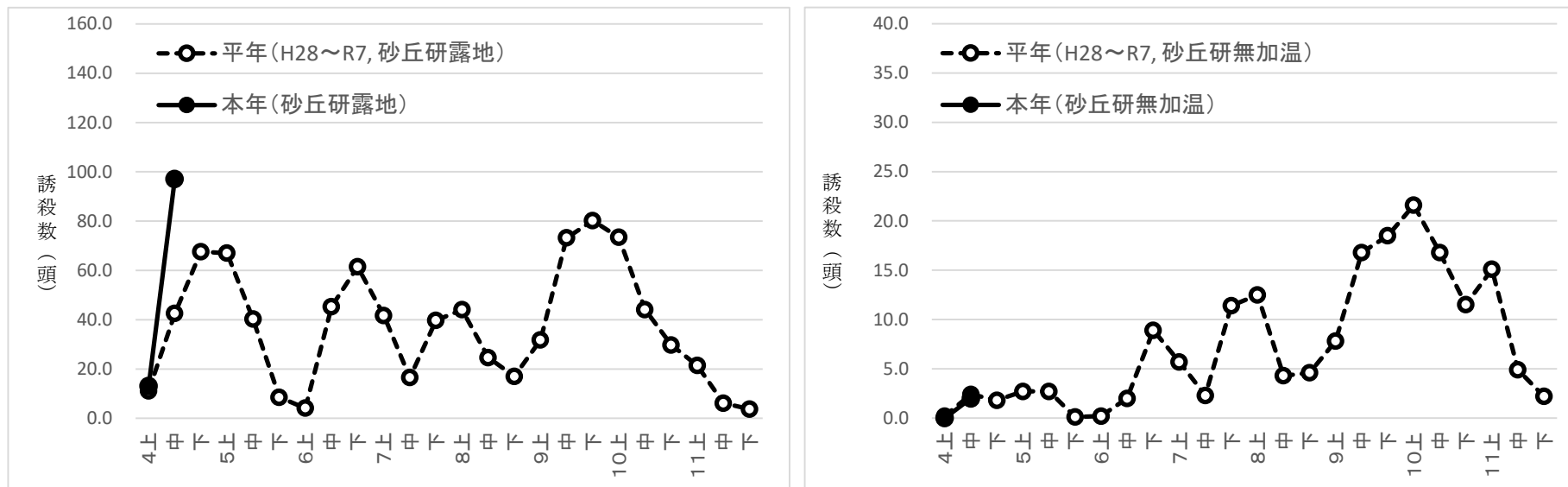
図1 フェロモントラップにおけるチャノコカクモンハマキの誘殺消長
