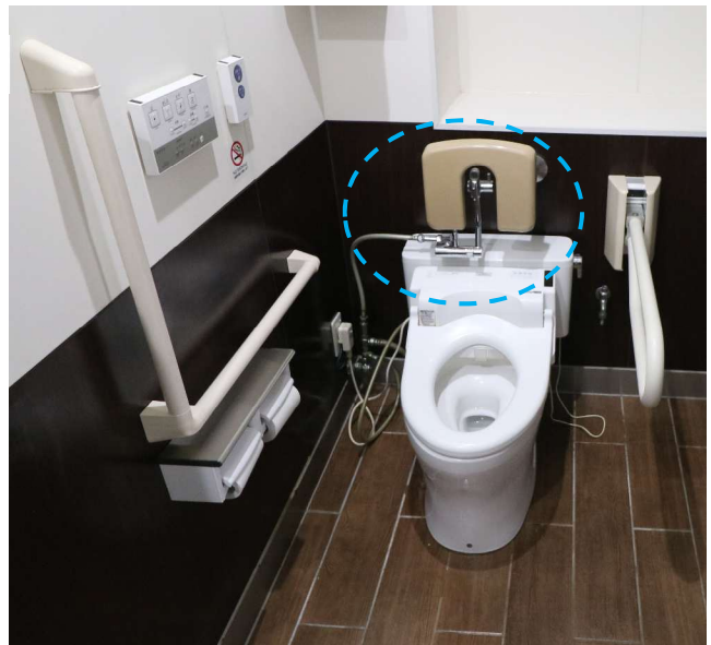
図 5 オストメイト用簡易型便房
