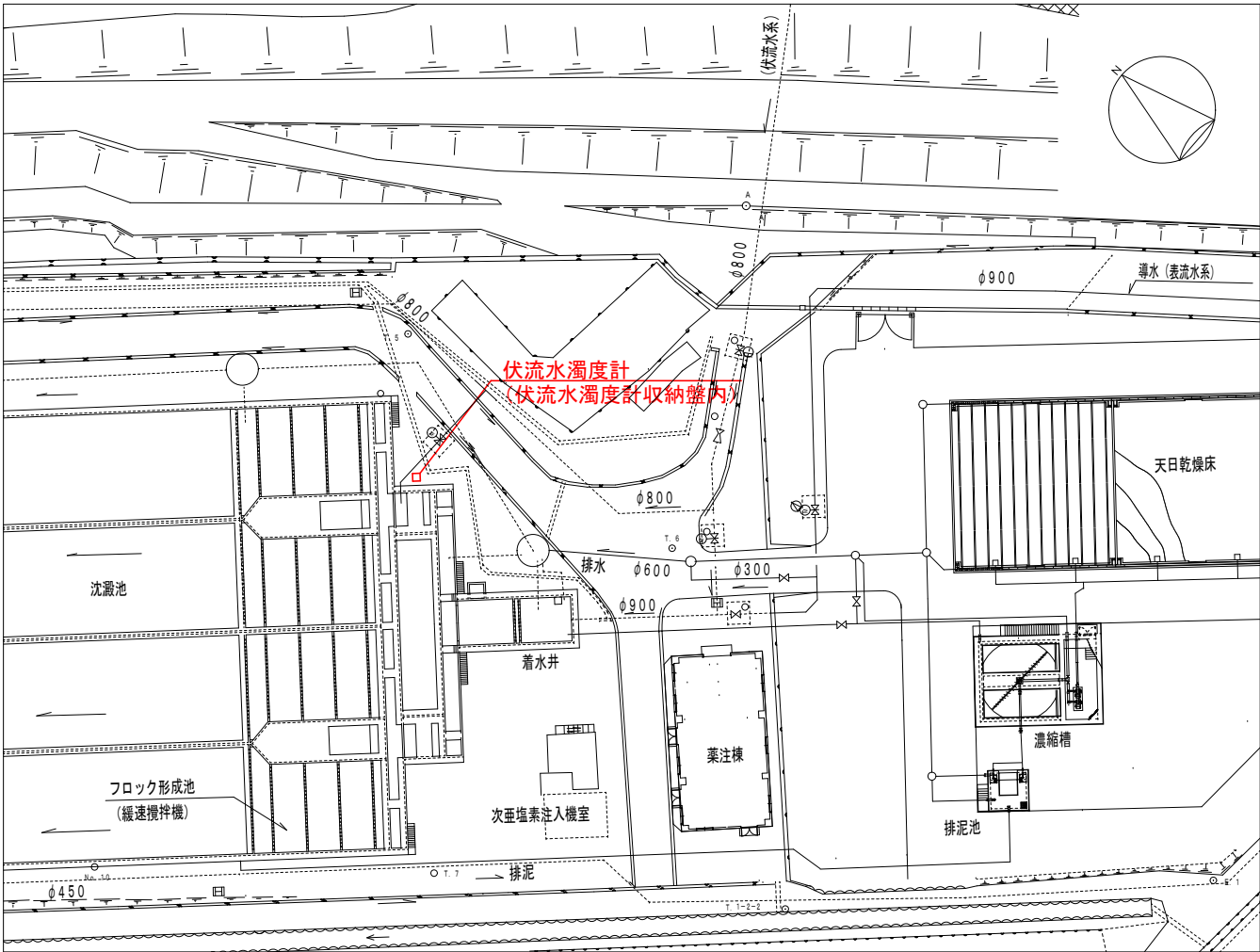
浄水場平面図
