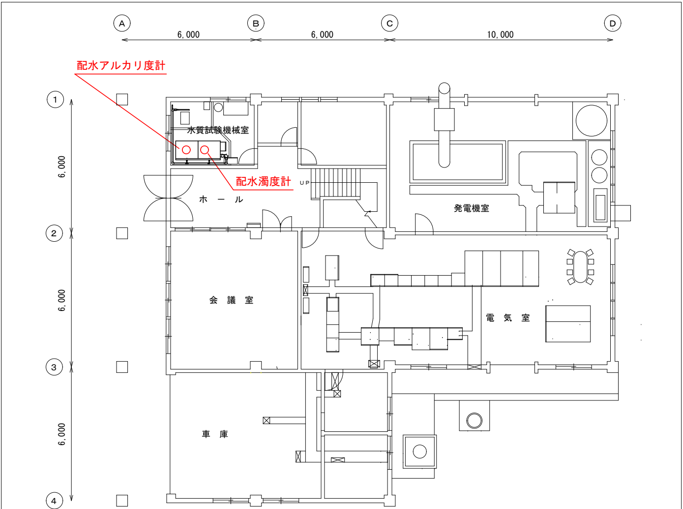
管理棟1階平面図
