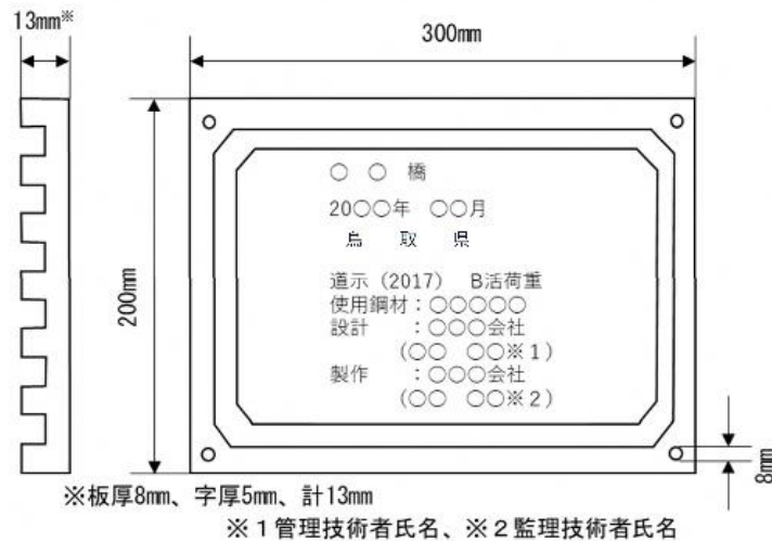
図3-2-2 銘板の寸法及び記載事項
