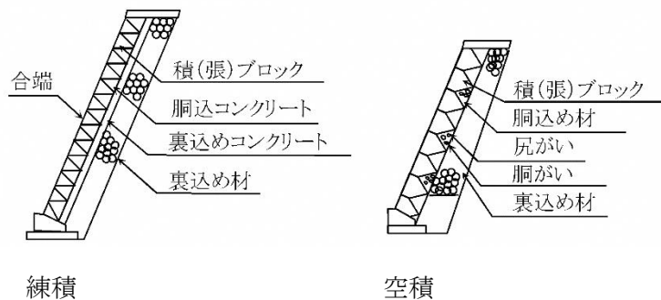
図3-2-5 コンクリートブロック工
