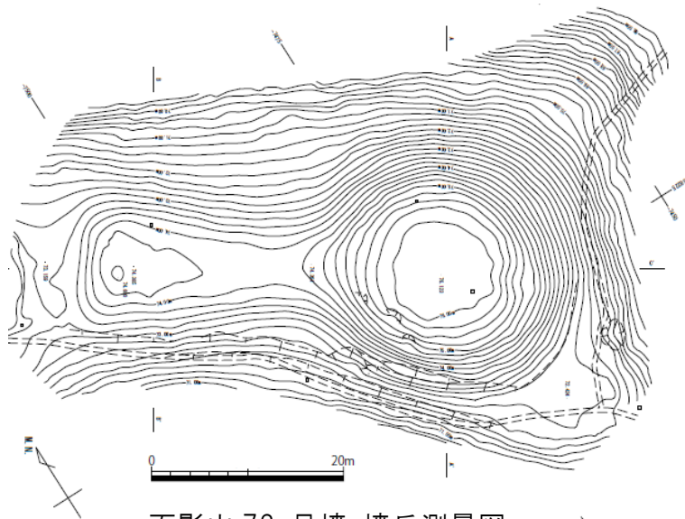
面影山73号墳 墳丘測量図
