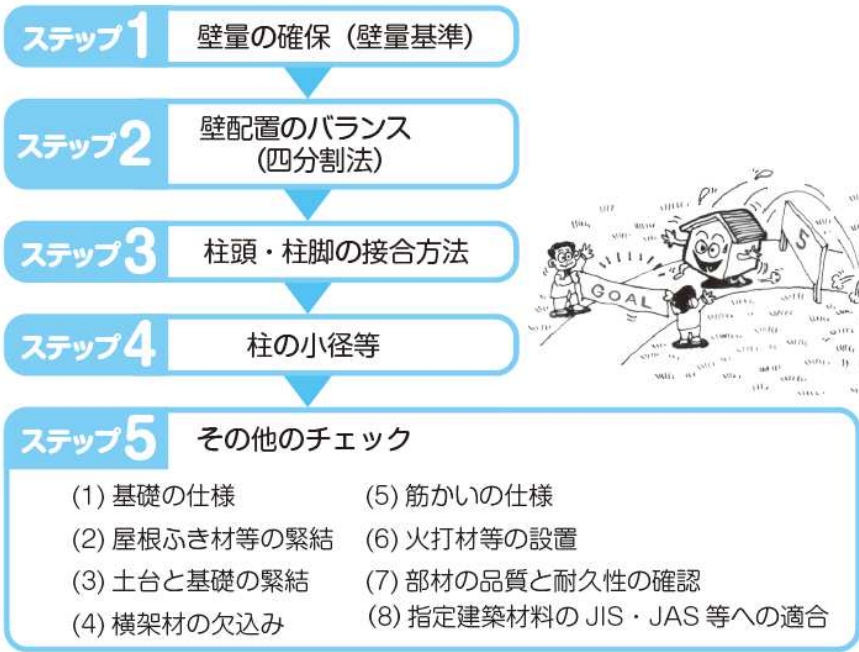
図 3 - 1 構造の安全性を確認する 5つのステップ
