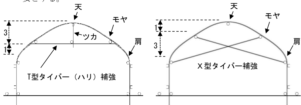
図3 T型タイバー、X型タイバーによる補強方法
