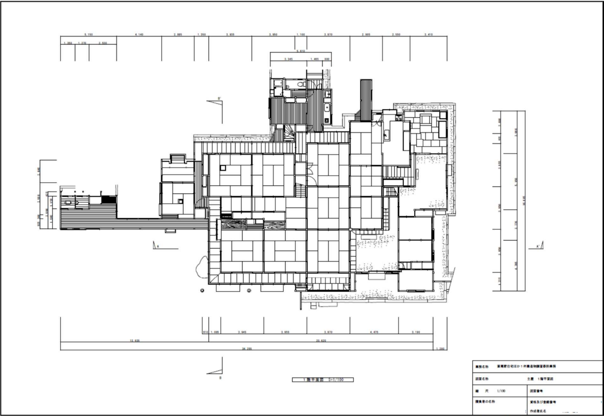
(図4) 成果品見本3 (平面図)
