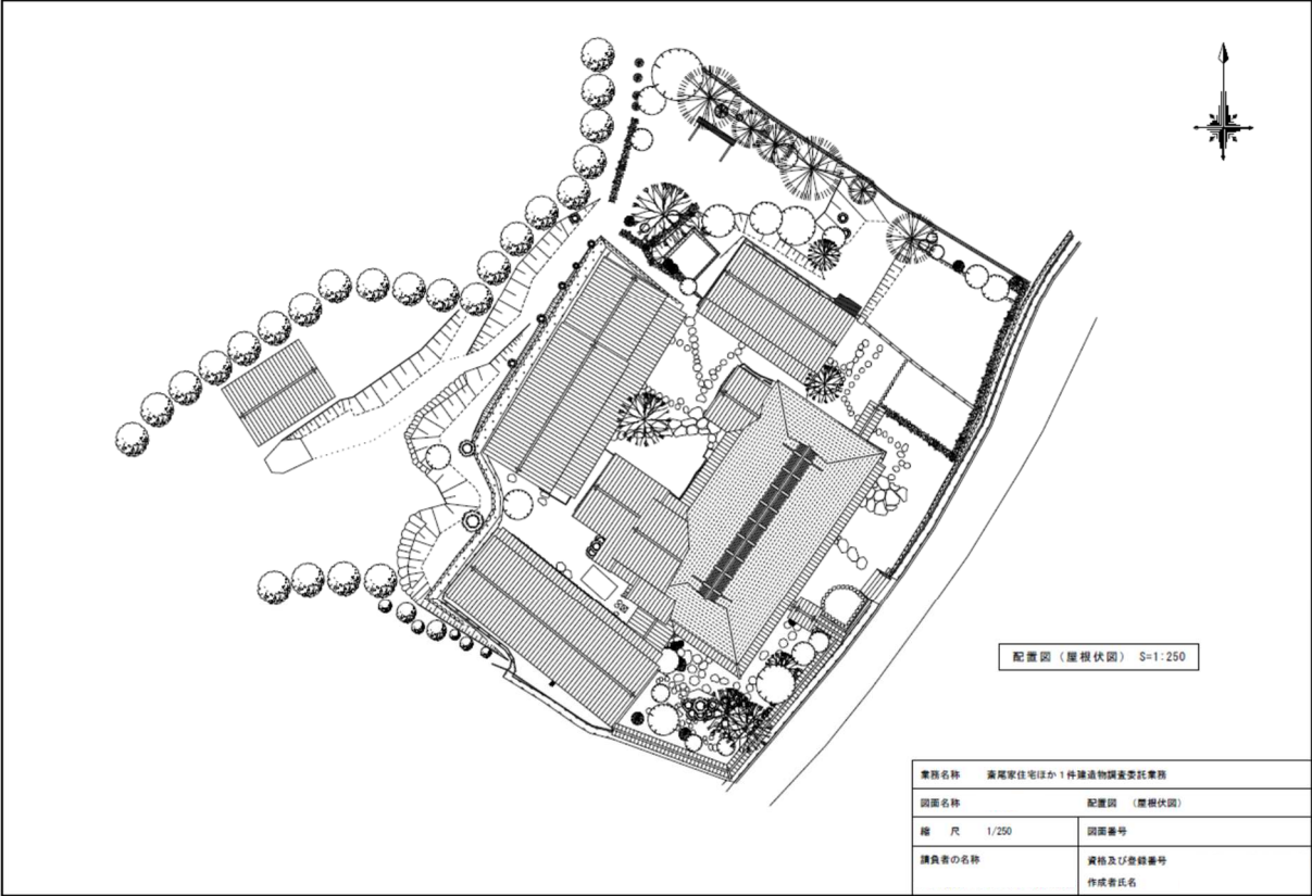
(図2) 成果品見本1 (配置図)
