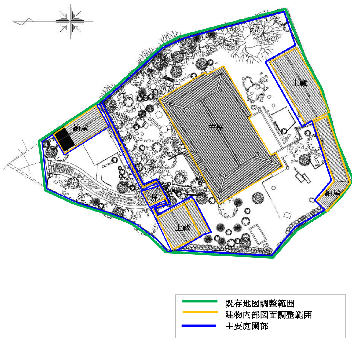
(図 2 - 3) 地図調整・測量範囲
