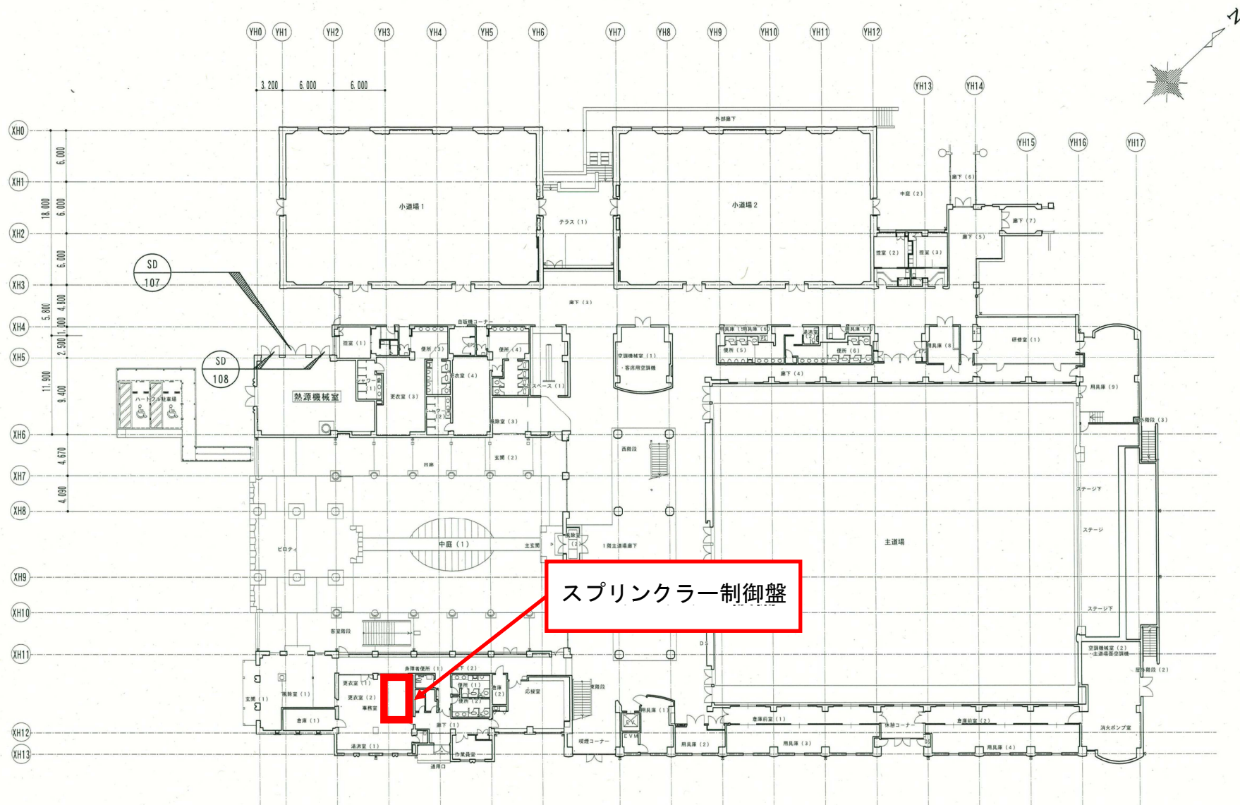
1階平面図 1:400
