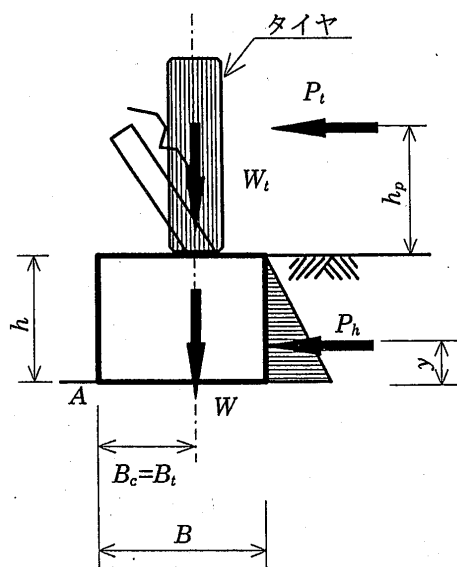
図 9-3-4 設計条件 [参 9-4 出典：公益社団法人日本道路協会 車両用防護柵標準仕様・同解説 p. 133]
