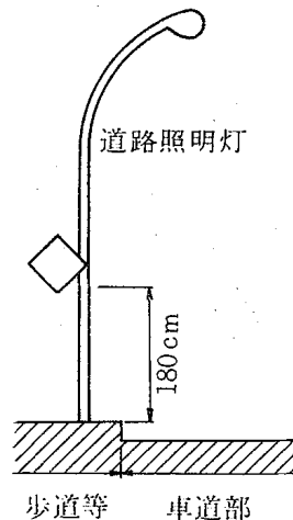
図 9-7-10 [参 9-6 出典：公益社団法人日本道路協会 道路標識設置基準・同解説 p. 66]
