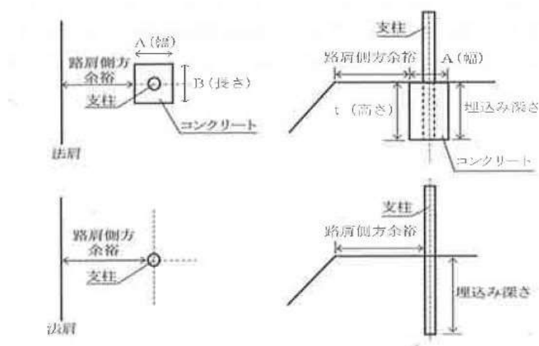
図 9-4-1 一般的な歩行者自転車用柵の支柱埋込み例
