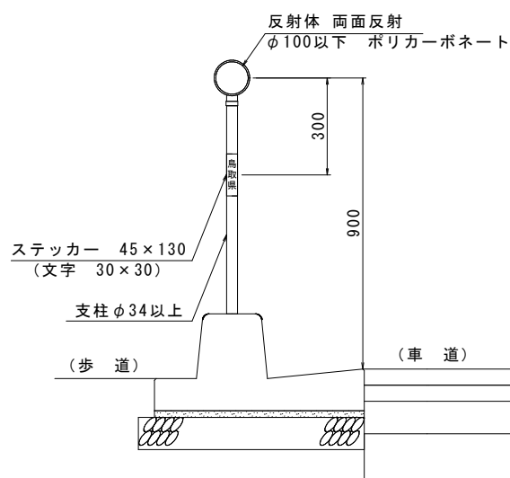
図 9-5-5 [参 9-16 鳥取県県土整備部 小構造物標準設計図集 P6-5]
