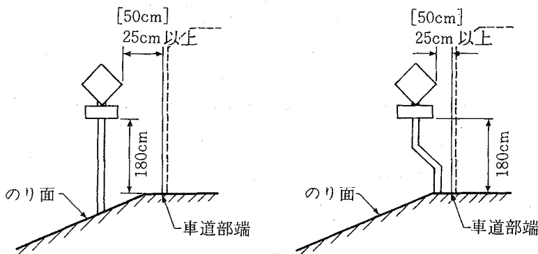
図 9-7-3 [参 9-6 出典：公益社団法人日本道路協会 道路標識設置基準・同解説 p. 63]
