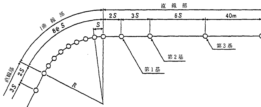
遷移地点における視線誘導標の設置間隔
