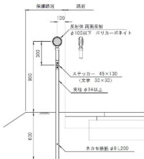
図 9-5-5 [参 9-16 鳥取県県土整備部 小構造物標準設計図集 P6-5]
