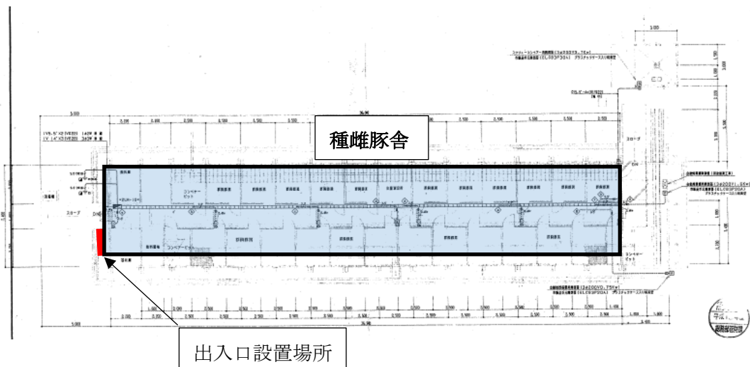
4 種雌豚舎平面図
