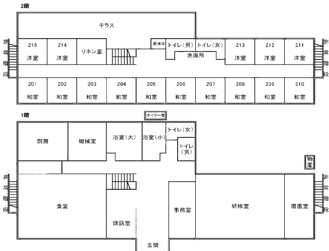
鳥取市サイクリングターミナル 砂丘の家平面図
