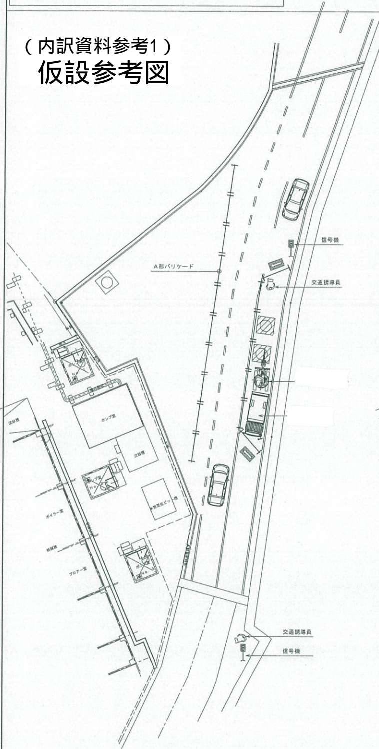
町道部 仮設図 (1) S=1/200
