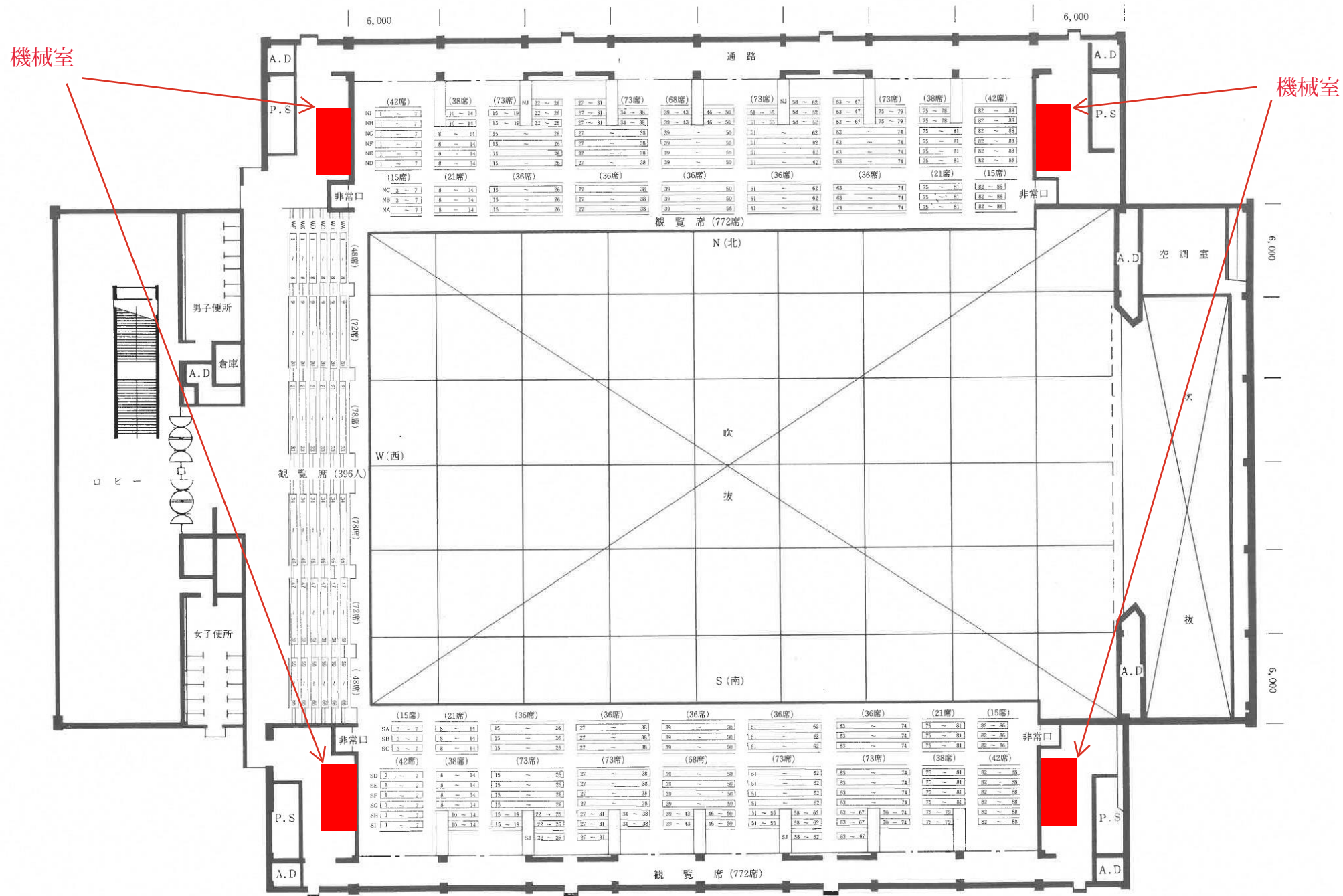
鳥取産業体育館二階平面図
