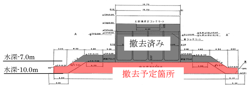
横断面図
