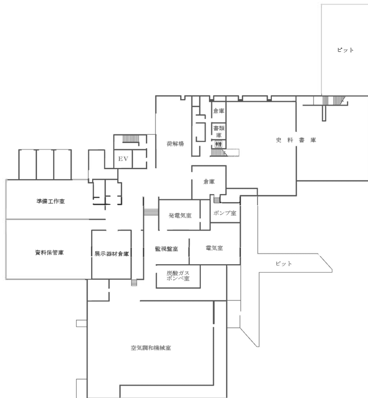
地階平面図
