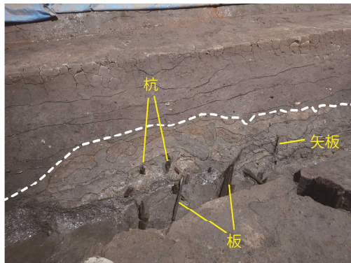
杭や板によって補強された盛土の土層断面 (白破線：確認した盛土の形) ※中心域：青谷上寺地遺跡で、弥生人の活動の中心となっていた微高地
