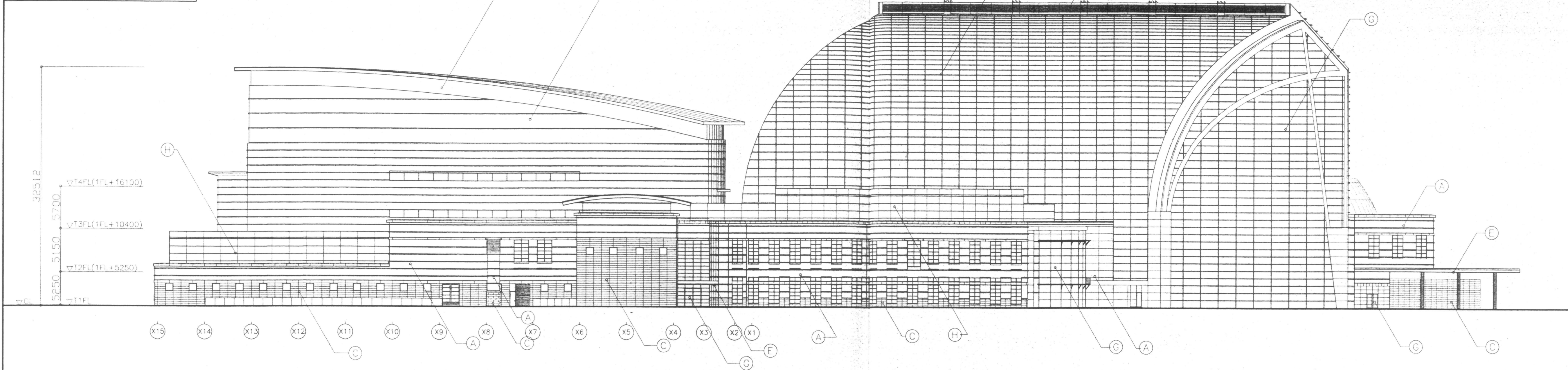
北立面図 1/300
