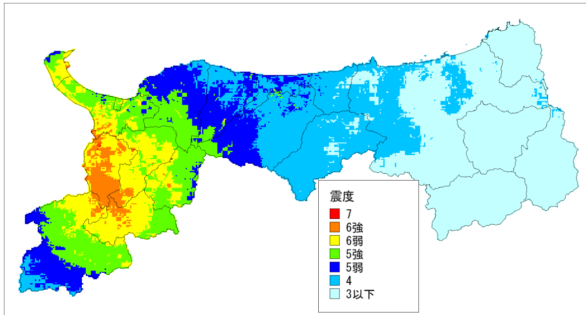
図4-3 (1) 鳥取県西部地震断層の震度分布
