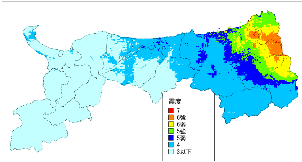
図4－5（1） 雨滝－釜戸断層の震度分布
