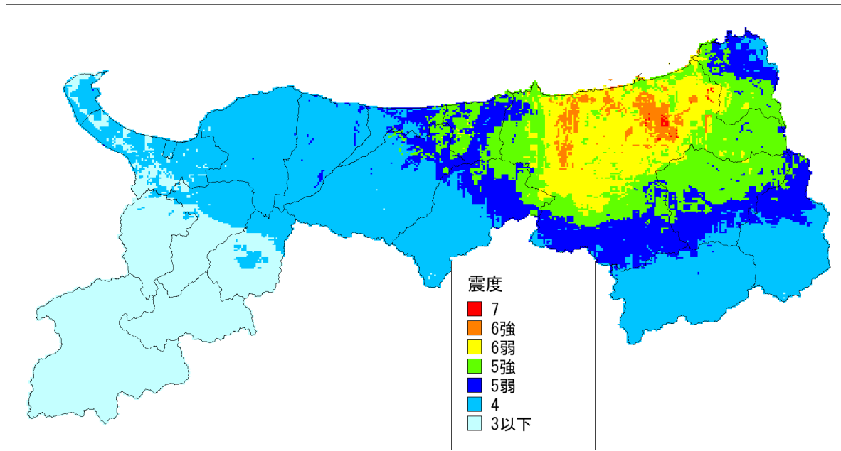
図4-1 (1) 鹿野・吉岡断層の震度分布
