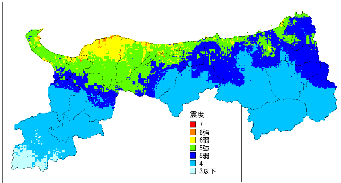
図4-4 (1) F55 断層の震度分布
