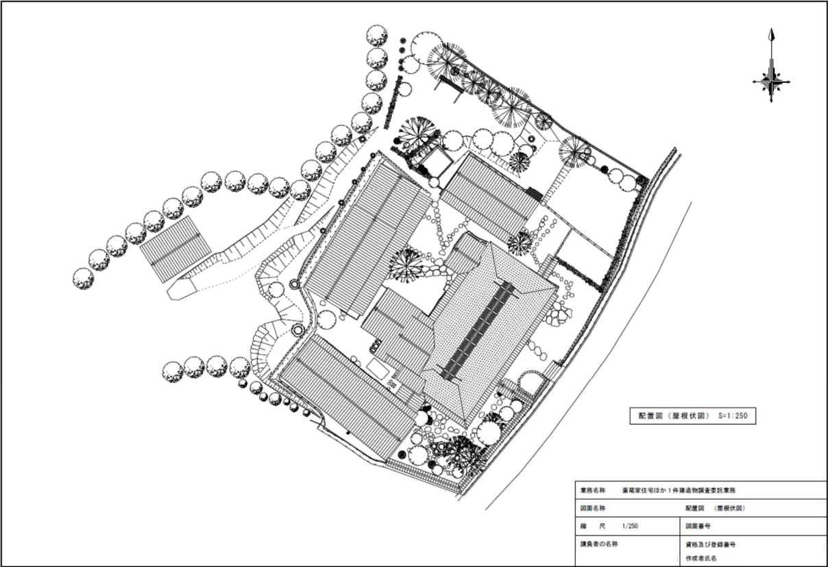
(図5) 成果品見本1 (配置図)
