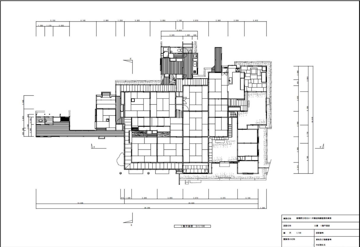
(図6) 成果品見本2 (平面図)
