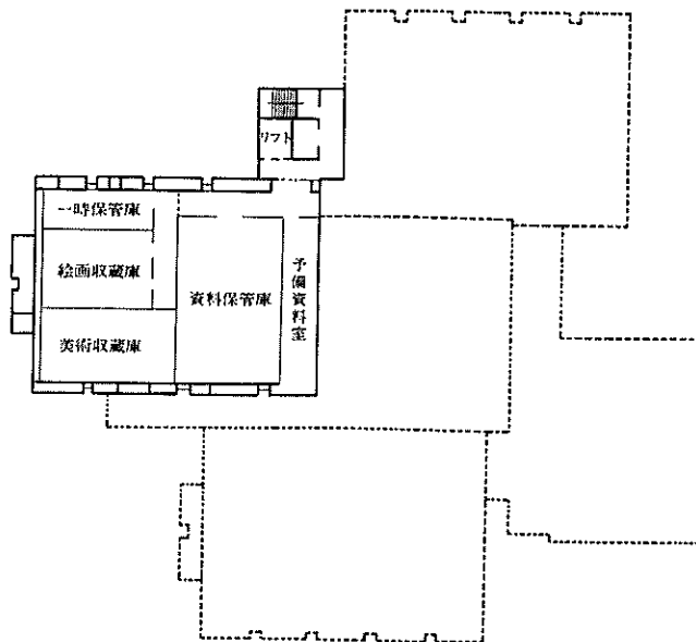
屋階平面図
