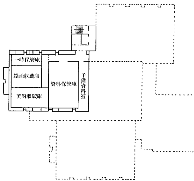
屋階平面図
