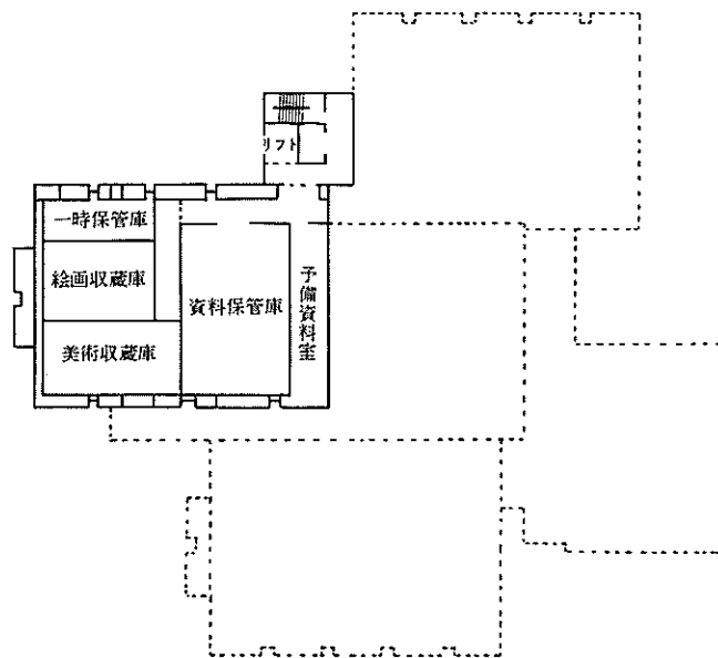
屋 階 平 面 図
