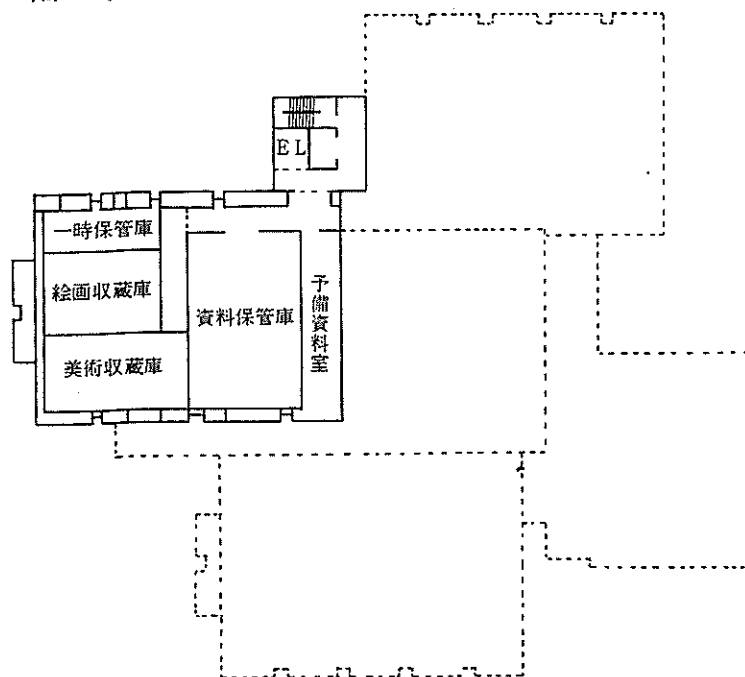
屋階平面図
