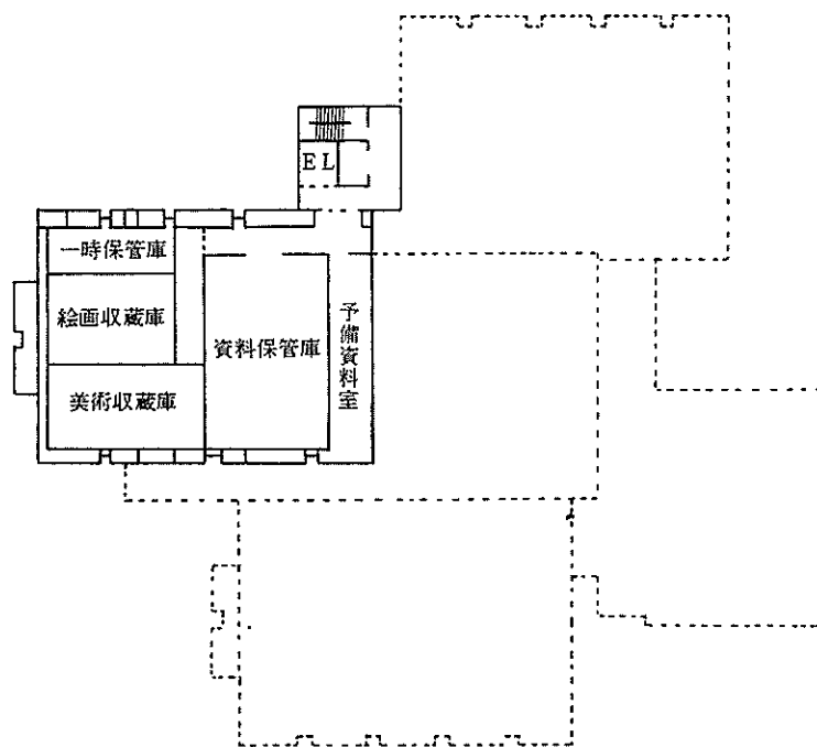
屋階平面図
