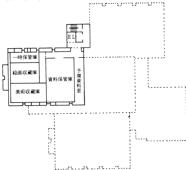
屋 階 平 面 図
