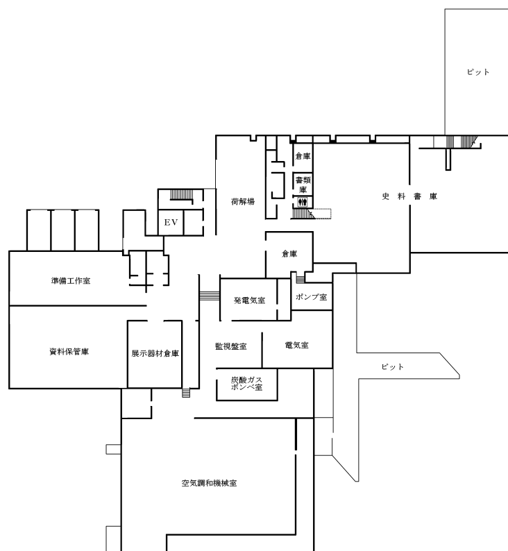
地階平面図
